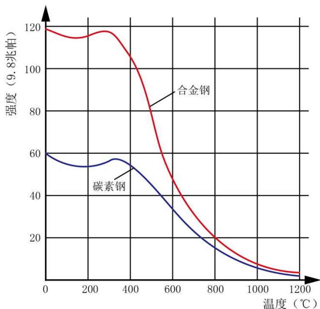
钢的高温强度变化曲线
